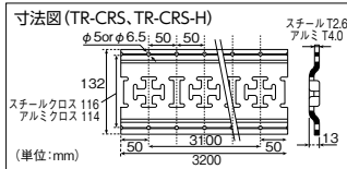
TR-CRS-H (クロス・ビス穴あり)
