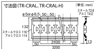
TR-CRAL-H (クロス・ビス穴あり)
